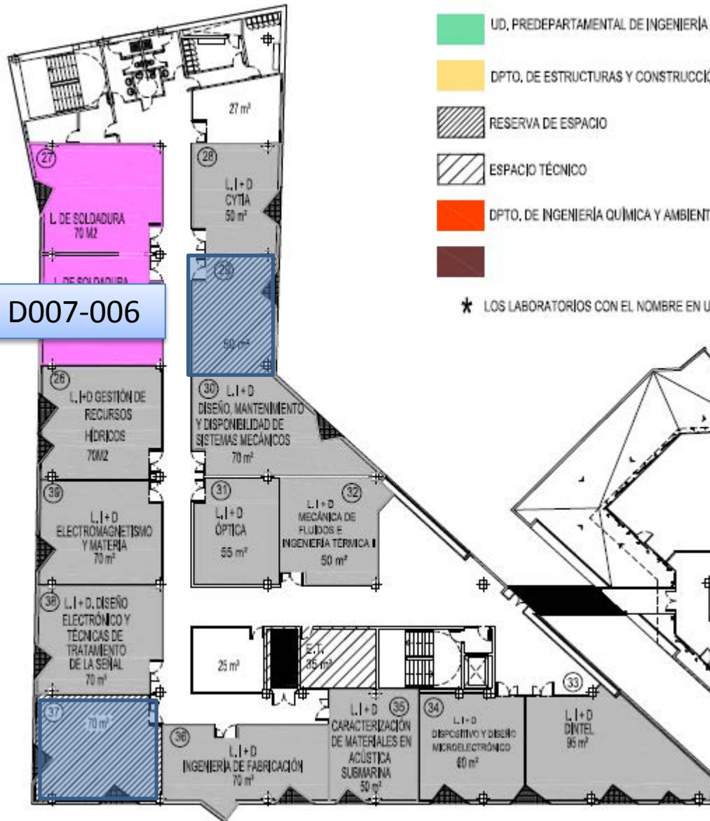
PLANTA 3º
