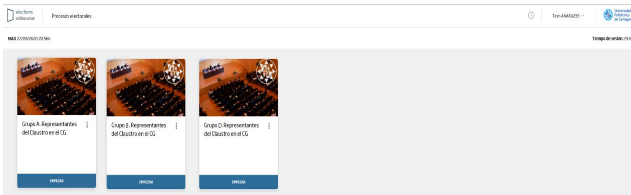
Figura 1. Pantalla inicial.
